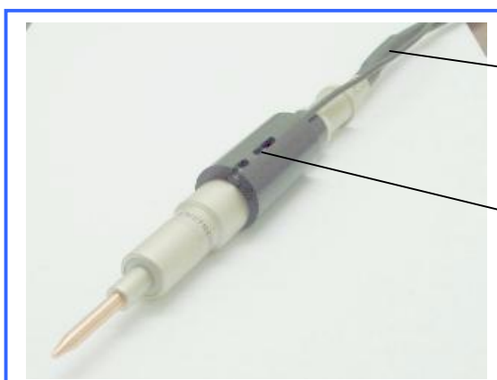
gefederter Elektrodenhalter
